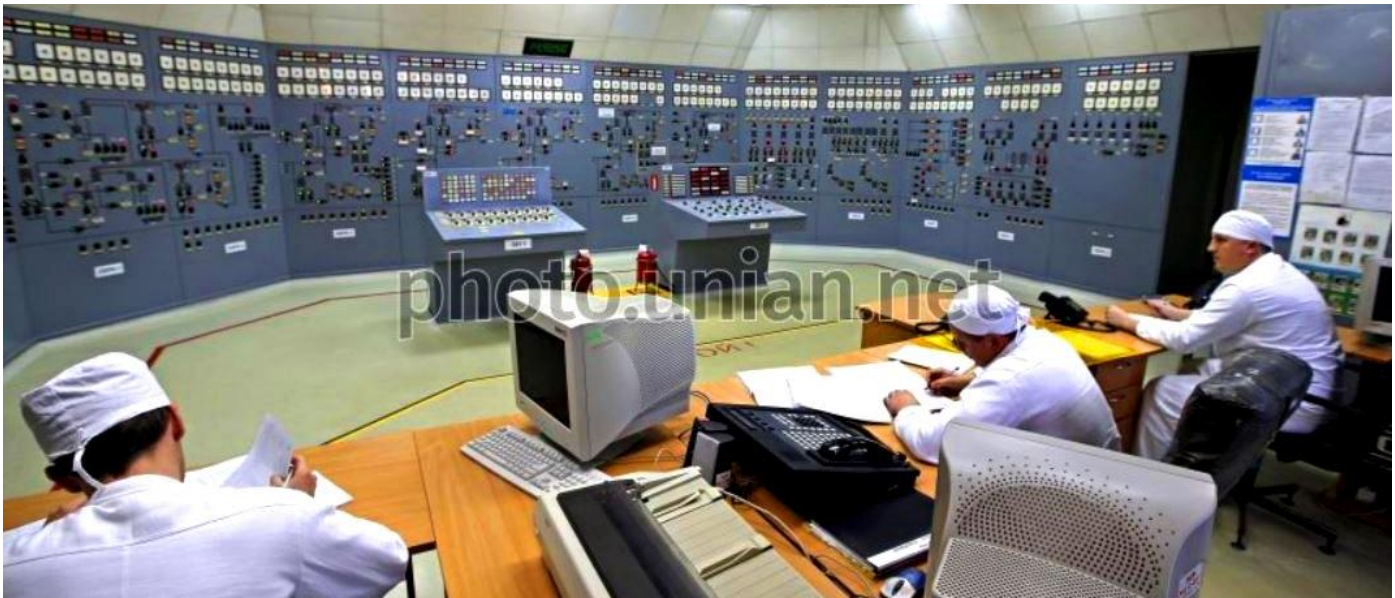
Salle de contrôle-commande de Zaporijia.
